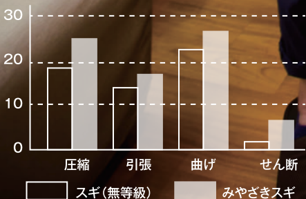
●みやざきスギの強度と無等級スギの基準強度(単位:N/mm)
